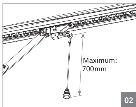
Position 01 • Moteur verrouillé Position 02 • Moteur déverrouillé
