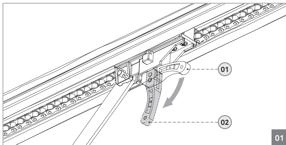
Position 01 • Moteur verrouillé Position 02 • Moteur déverrouillé
